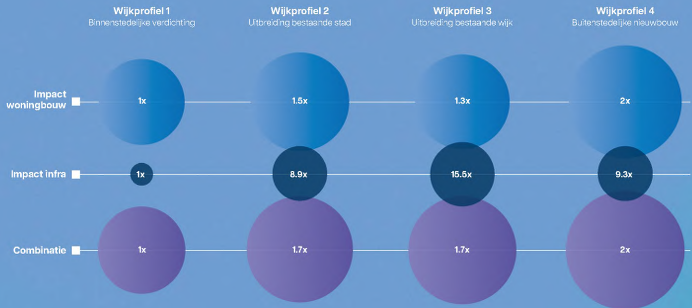
Abbeelding 51. De CO 2 -impact verschilt aanzienlijk, afhankelijk van de locatie waar wordt gebouwd. Bron: LEVS, Copper8, Metabolic (2025) CO 2 -impact van woningbouwlocaties.
