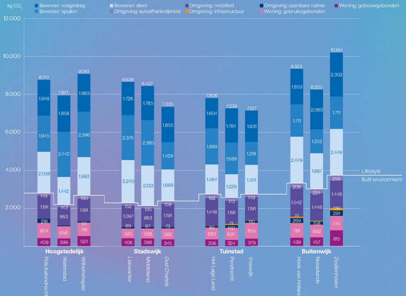
Abbeelding 52. De totale CO 2 -uitstoot (per persoon, per jaar) per type stadswijk is het hoogst voor de uitbereidingswijken. Met name de gebouwgebonden uitstoot is hier hoog. Bij tuindorpen is de gebruikersuitstoot lager, voor de compactere stadswijken is dit het geval voor de gebouwgebonden uitstoot. Bron: PosadMaxwan, Cityföörster, Gemeente Rotterdam (2025) Carbon based urbanism.
