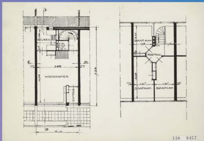
Afbeelding 20. Plattegrond van woningen in de wijk Kiefhoek gebouwd naar het ontwerp van de architect J.J.P. Oud. Bron: Rijksvoorlichtingsdienst (RVD), bestandnr. 130-0457, Nationaal Archief.
