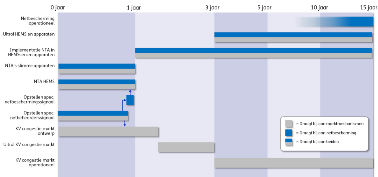
Figuur 6.1: Technisch ontwikkelpad KV-netbescherming
