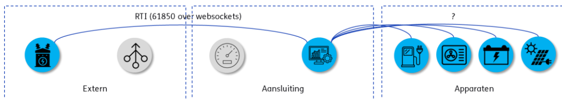
Figuur 4.4: Real Time Interface v2 voor laagspanning
